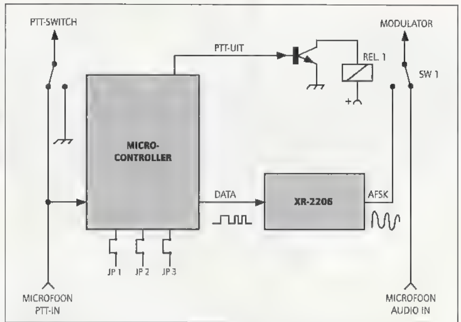
Figuur 6: Een blokschematische weergave van een ATIS-encoder.
